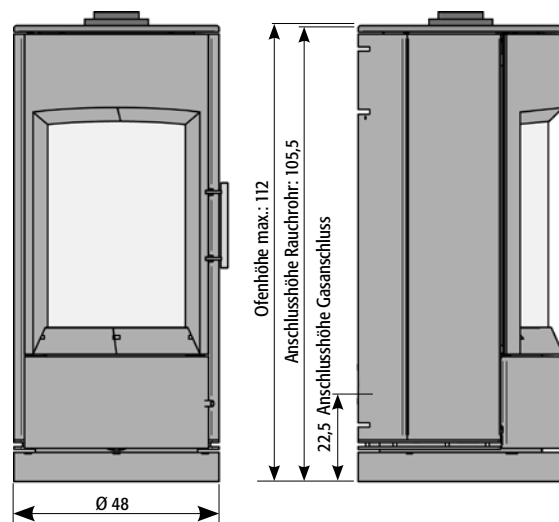
Vorderansicht
